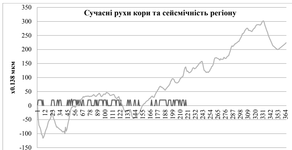
Рис. 6. Сучасні рухи кори в зоні Оаиського глибинного розлому (крива сірого кольору), місцева сейсмічність (крива чорного кольору). 2021 рік. Закарпатський внутрішній прогин
